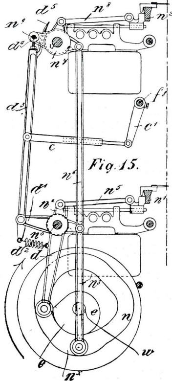
Festonapparat, Patent No. 12 798, mit Antupfen der Sticknadel an den Stoff. Damit wurde der Knopfstich möglich.
