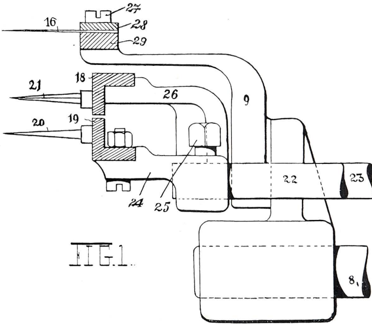
Bohr- und Stüpfelapparat für Schifflistickmaschinen (⊕ Patent No. 33 207).
