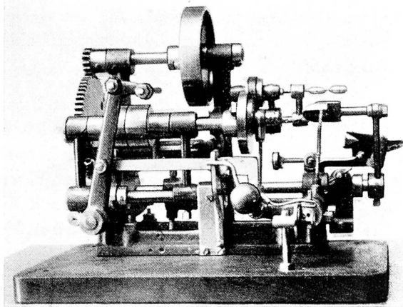
Bobinenmaschine mit zwei Bobinen auf einem Dorn. ⚙ Patent No. 5349
