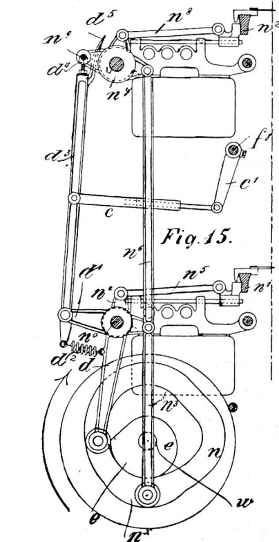
Festonapparat, Patent No. 12 798, mit Antupfen der Sticknadel an den Stoff. Damit wurde der Knopfstich möglich.
