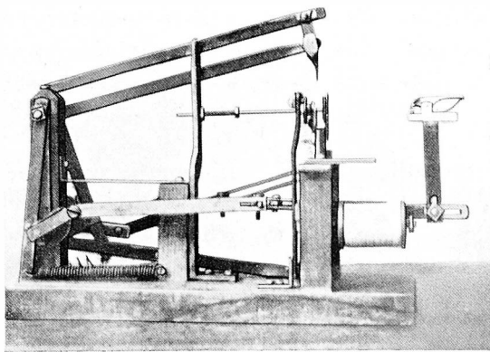
Einfüdelmaschine, Modell 1884, ⚙ Patent No. 25. Die Handkurbel befindet sich verdeckt auf der andern Seite. Eine Umdrehung zieht den Faden durchs Nadelöhr und verknotet ihn.
